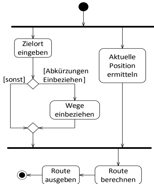
Abbildung 3: Beispiel eines Aktivitätsdiagramms
